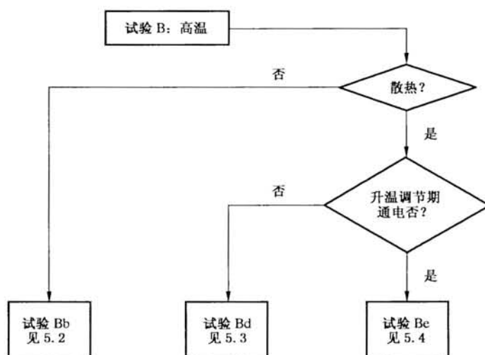
图 1 试验 B: 高温试验方框图
